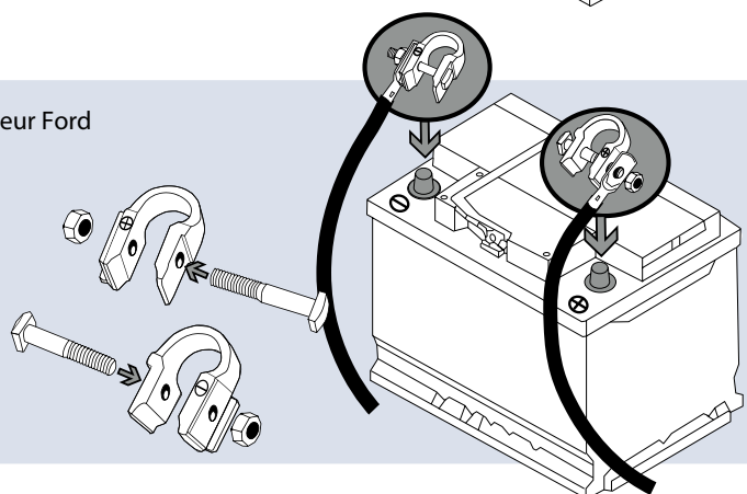
Adaptateur VW
